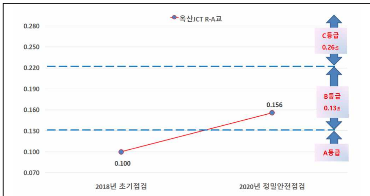
[그림 1.4.1] 옥산JCT R-A교 상태평가 결과 비교 그래프
