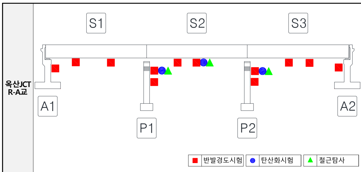
[그림 1.3.2] 비파괴시험 위치도
